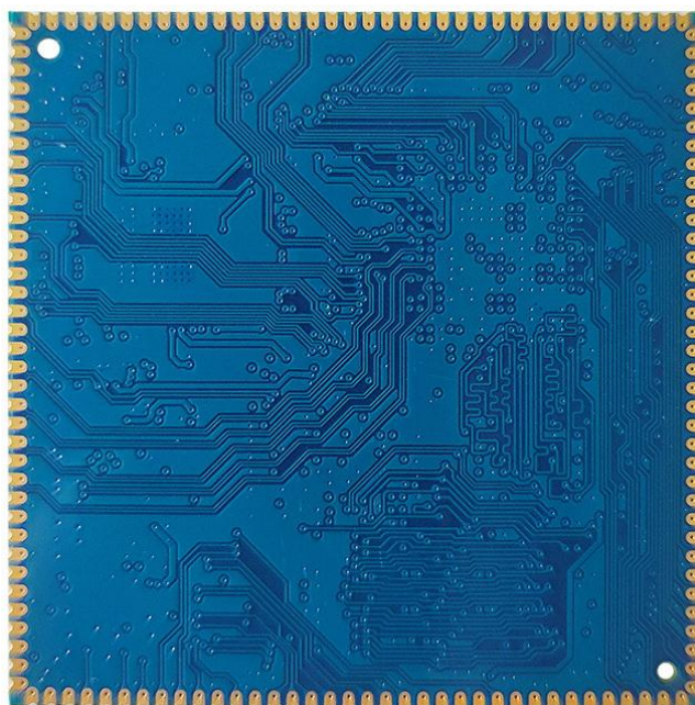
X30CV2 背面图
