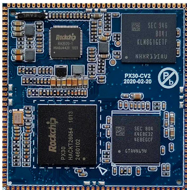
X30CV2 正面图
